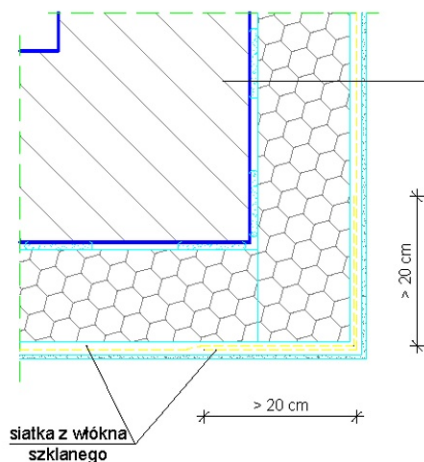
Zbrojenie narożnika podwójną siatką z włókna szklanego
