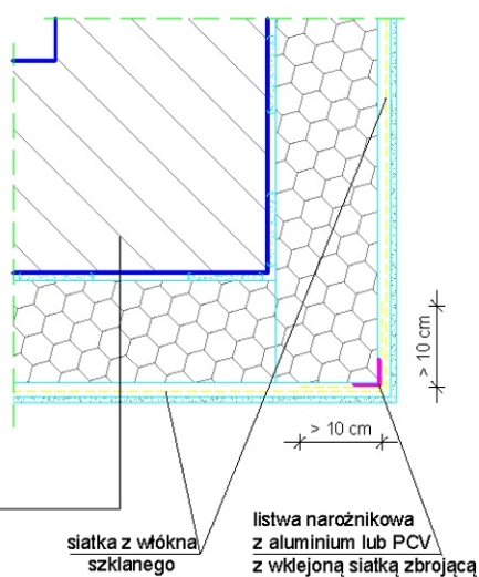
Zbrojenie narożnika listwą narożnikową z siatką
