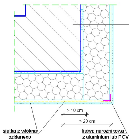
Zbrojenie narożnika listwą narożnikową
