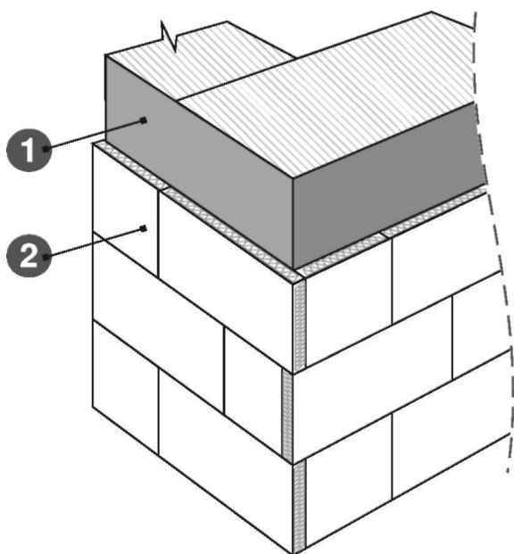
rys. 4. Układ płyt styropianowych przy narożniku budynku.
